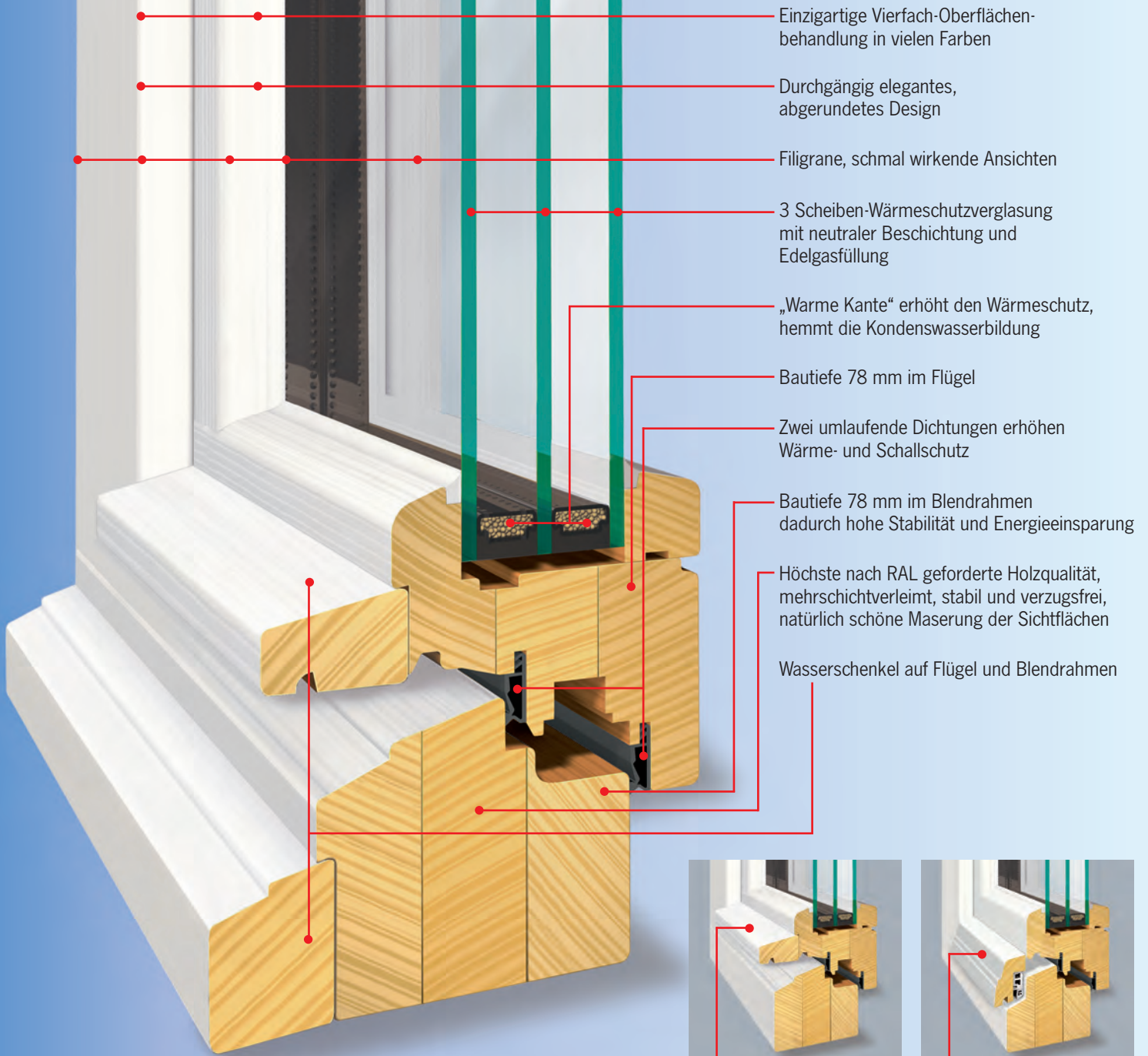
Optional: Wasserschenkel auf Flügel
