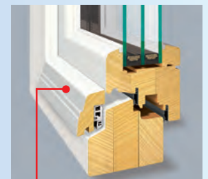
Optional: Abgedeckte Regenschiene durch Profileiste
